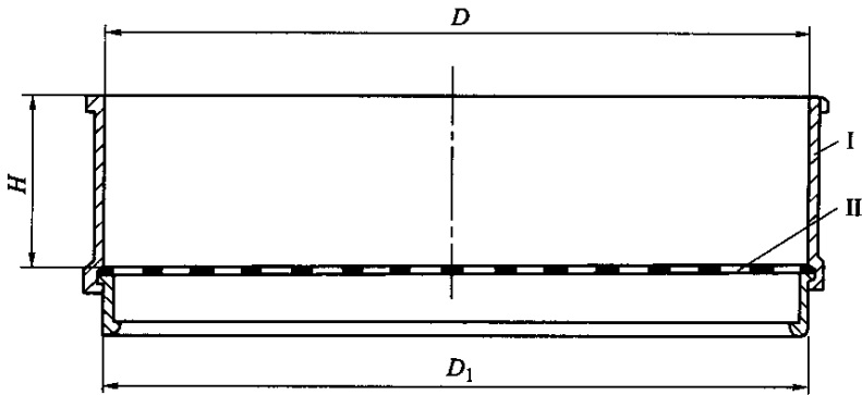
图 A-1 标准筛的筛框(I-筛框;II-筛面)
