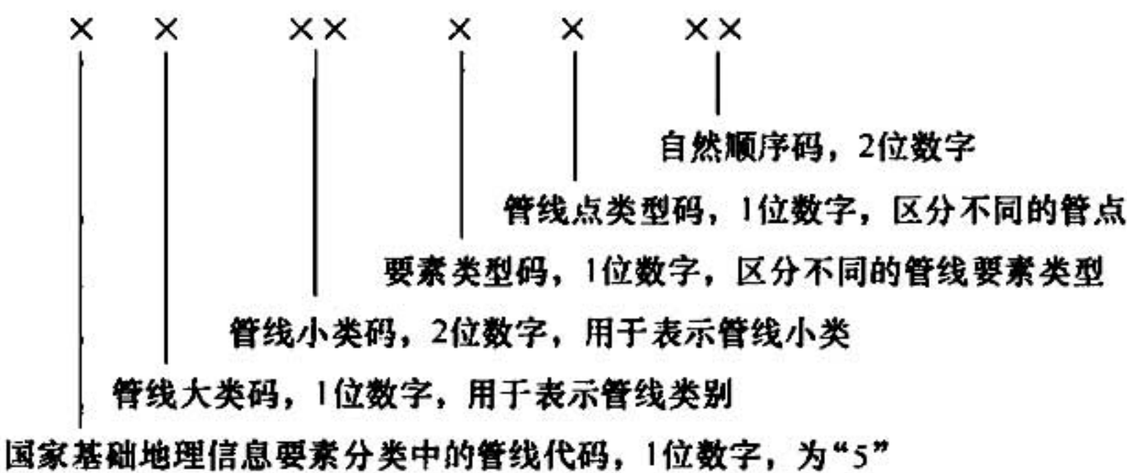
图 7.2.5 管线要素编码结构
