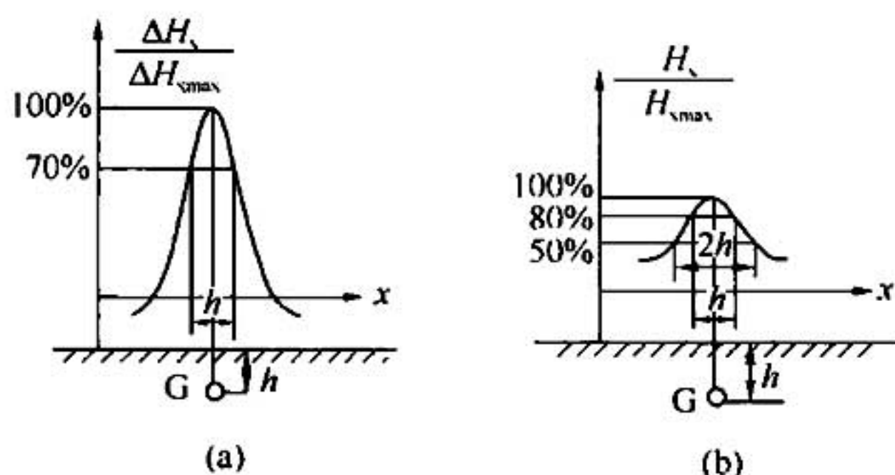
图 2 电磁感应法管线定深示意
