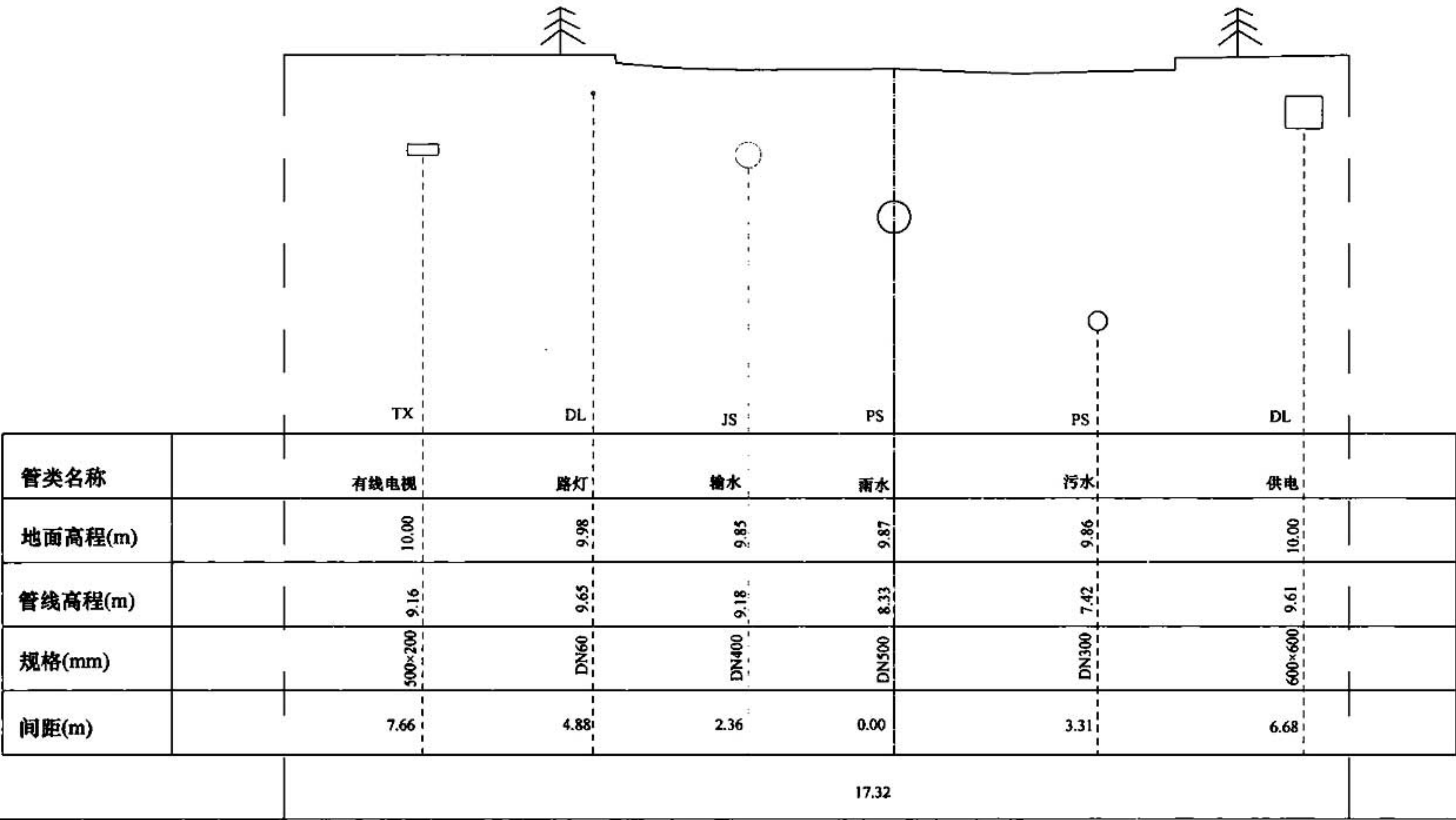
图 J-3 管线横断面图样
