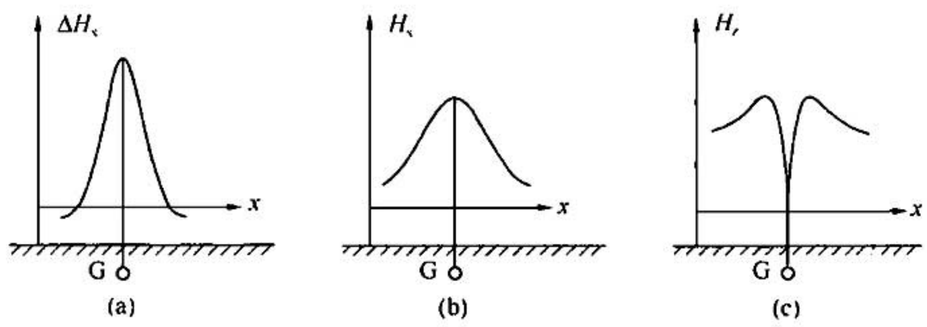
图 1 电磁感应法管线定位示意
