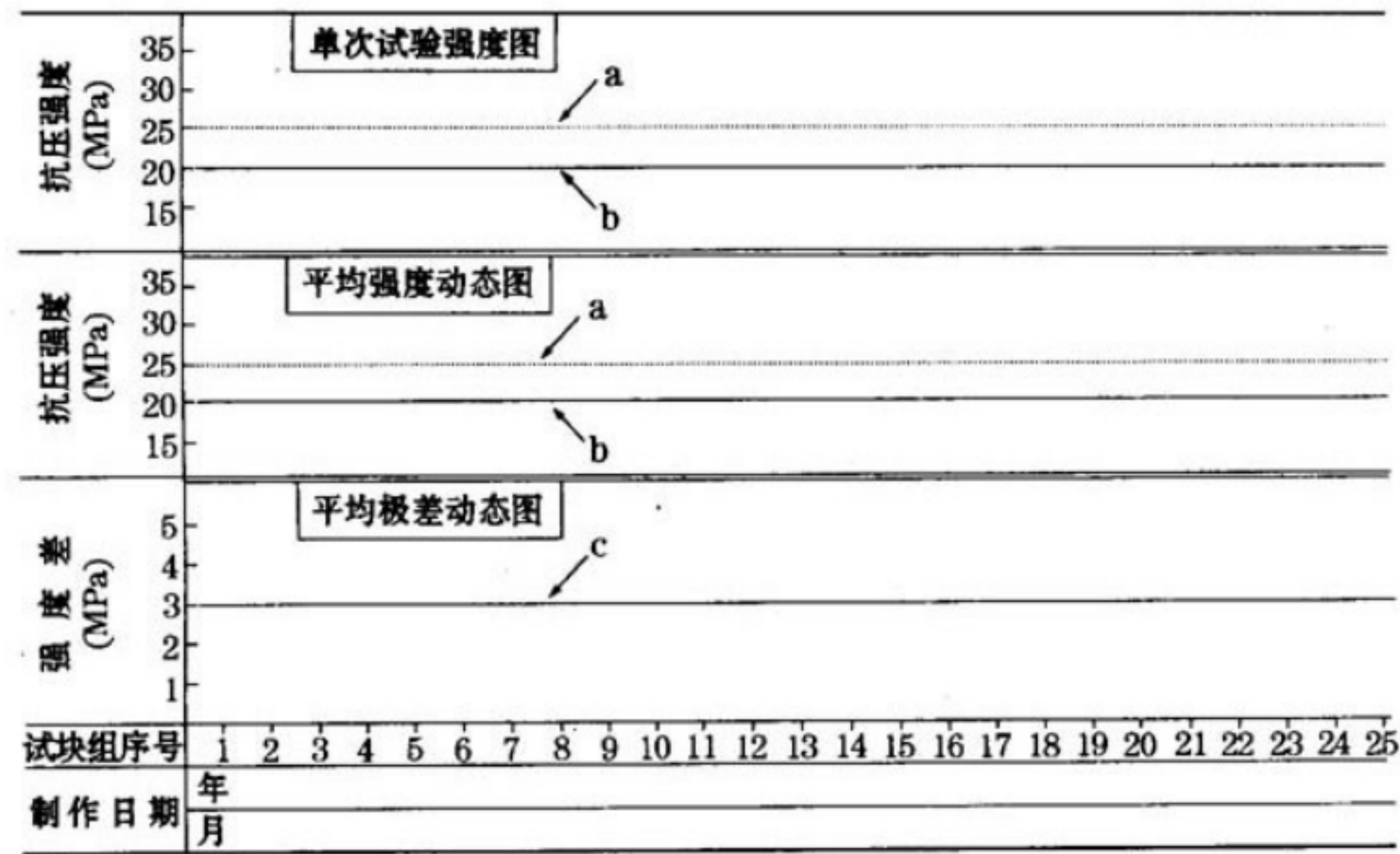
图 D 喷射混凝土强度质量控制图
