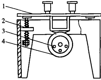
图 T0506-2 代用胶砂振动台 1-台面;2-弹簧;3-偏重轮;4-电动机
