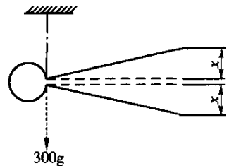
图 T0505-3 雷氏夹受力示意图
