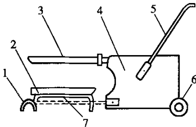
图 T0563-1 两用机筛分工作状态
