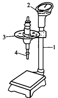
图 T0527-1 贯入阻力仪示意图 1-主体;2-刻度盘;3-手轮;4-测针
