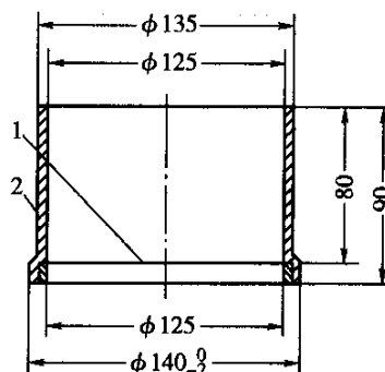
图 T0502-2 水筛(尺寸单位:mm) 1.筛网;2.筛框
