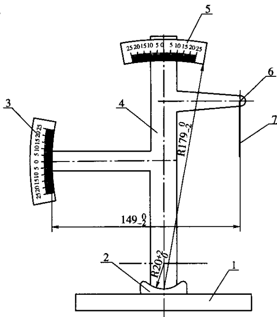
图 T0505-4 雷氏膨胀值测定仪(尺寸单位:mm)
