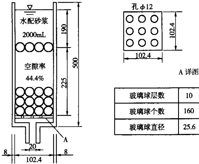
图 T0509-1 砂浆筒球流动仪示意图(尺寸单位:mm)
