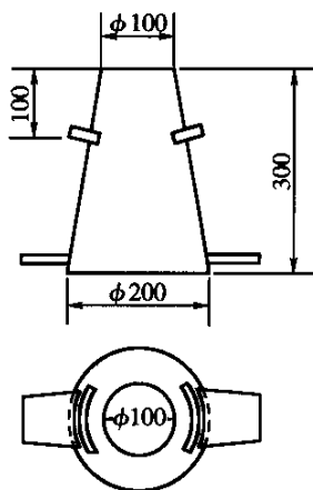
图 T0522-1 坍落度试验用坍落筒 (尺寸单位: mm)
