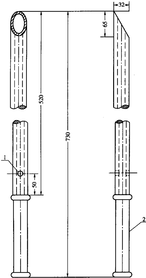
图 T0501-1 袋装水泥取样管(尺寸单位:mm) 1-气孔;2-手柄
