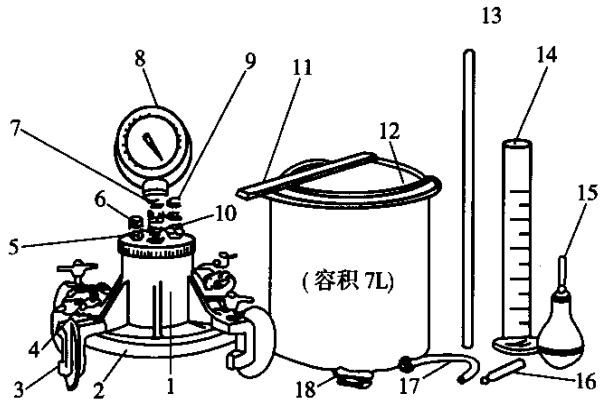
图 T0526-1 混合式气压法含气量测定仪
