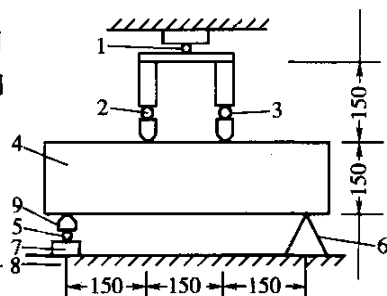
图 T0558-1 抗弯拉试验装置
