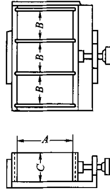
图 T0563-4 试模结构
