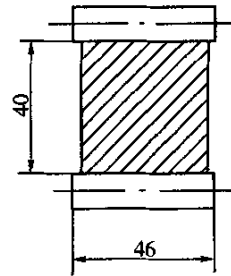
图 T0506-3 下料漏斗(尺寸单位:mm) 1-漏斗;2-模套
