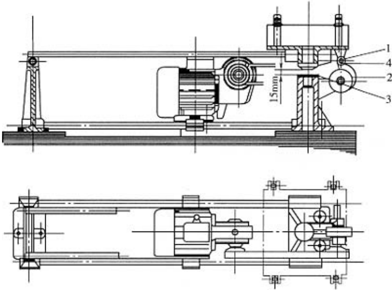
图 T0506-1 典型振实台
