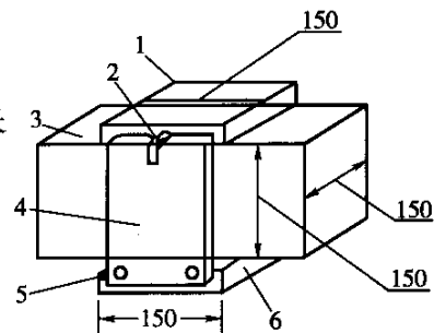
图 T0562-1 试件压板
