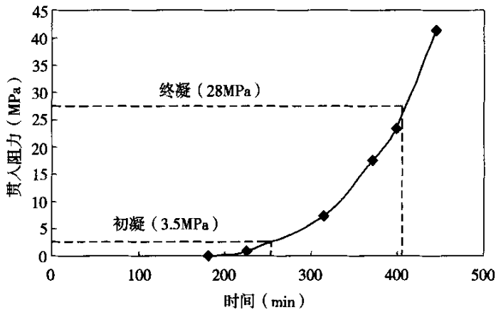
图 T0527-2 时间-贯入阻力曲线
