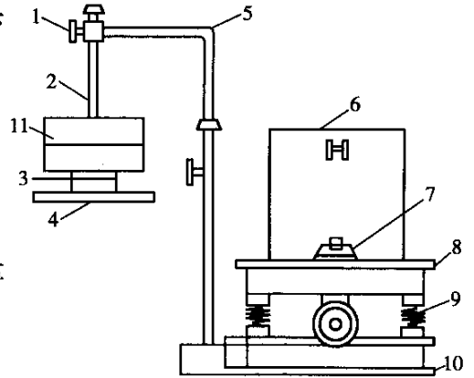
图 T0524-1 维勃工作度测定仪简图
