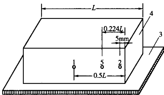
图 T0564-2 测示位置示意图
