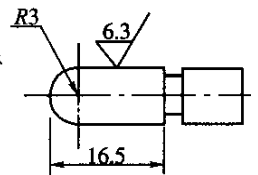
图 T0511-2 钉头 (尺寸单位:mm)
