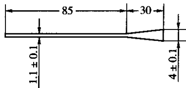
图 T0502-4 喷气嘴上开口 (尺寸单位:mm)
