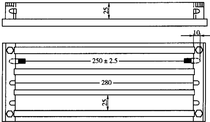
图 T0511-1 三联试模(尺寸单位:mm)
