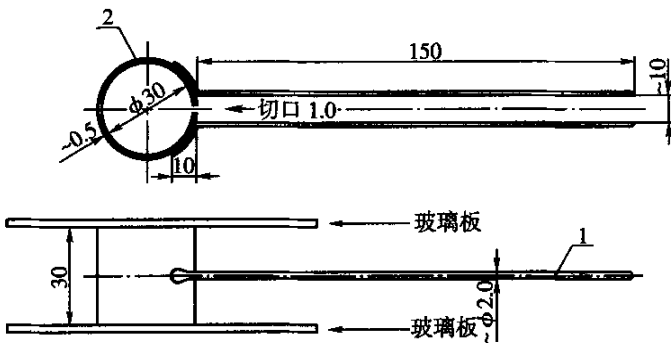
图 T0505-2 雷氏夹示意图(尺寸单位:mm)
