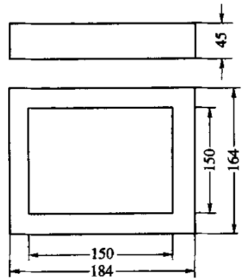
图 T0510-2 模套(尺寸单位:mm)
