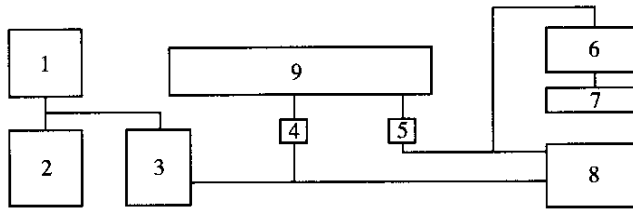
图 T0564-1 共振法混凝土动弹性模量测定工作原理图
