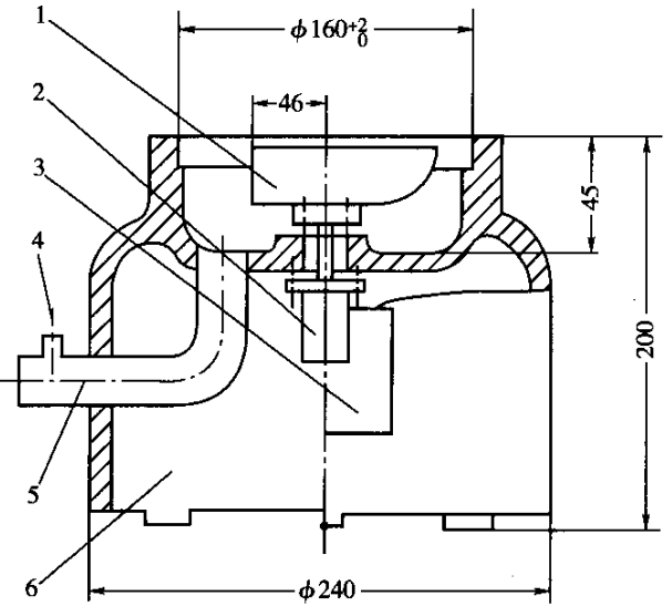
图 T0502-3 筛座(尺寸单位:mm)
