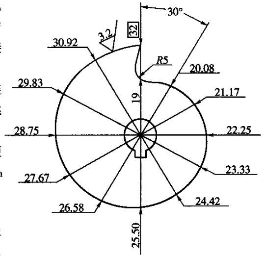
图 T0507A-2 凸轮示意图 (尺寸单位: mm)
