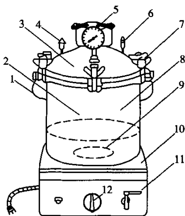
图 T0512-1 压蒸仪
