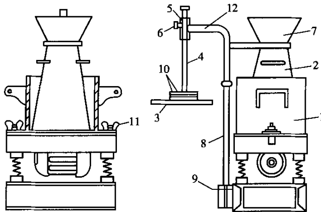
图 T0523-1 稠度计(维勃仪)
