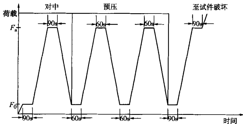
图 T0556-3 弹性模量加荷方法示意图
