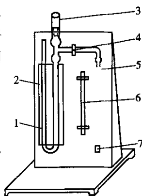
图 T0504-1 Blaine 透气仪示意图
