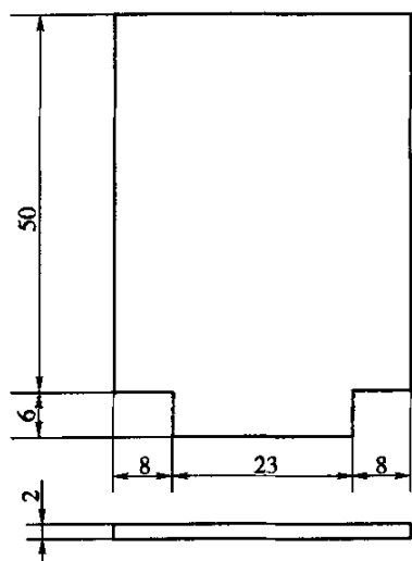
图 T0511-4 刮板(尺寸单位:mm)
