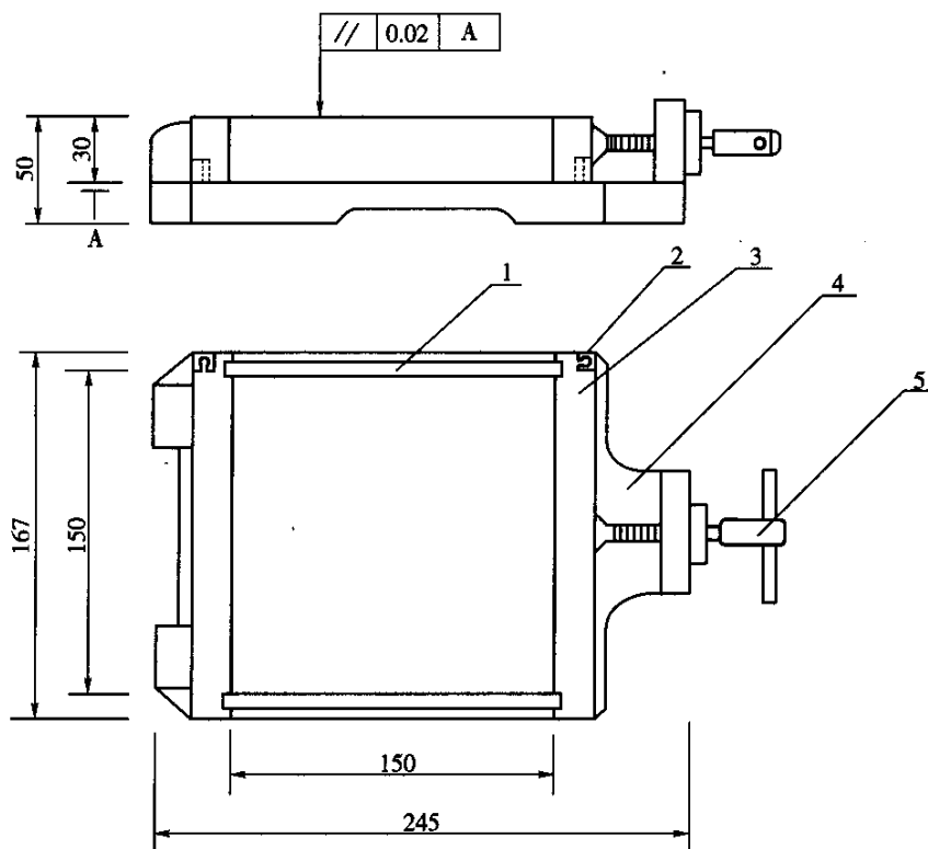
图 T0510-1 试模示意图(尺寸单位:mm)
