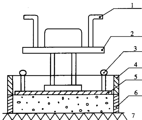
图 T0552-3 试件成型示意图
