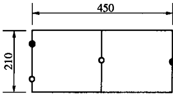
图 T0559-1 千分表架 (尺寸单位:mm)
