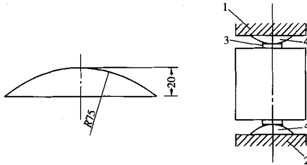
图 T0560-1 劈裂试验用钢垫条(尺寸单位:mm)
