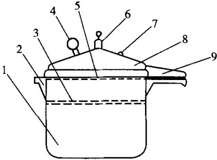
图 T0563-3 专用压蒸仪结构
