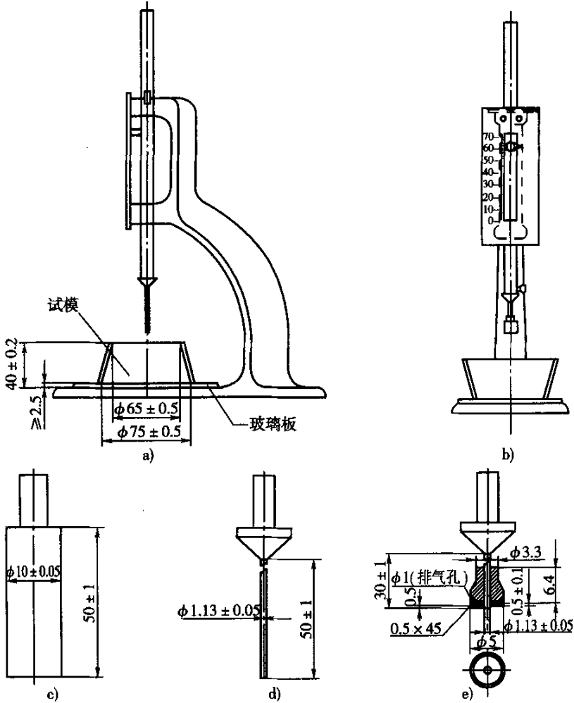
图 T0505-1 测定水泥标准稠度和凝结时间用的维卡仪(尺寸单位:mm)
