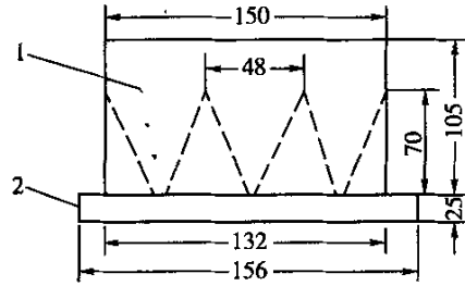
图 T0506-3 下料漏斗(尺寸单位:mm) 1-漏斗;2-模套
