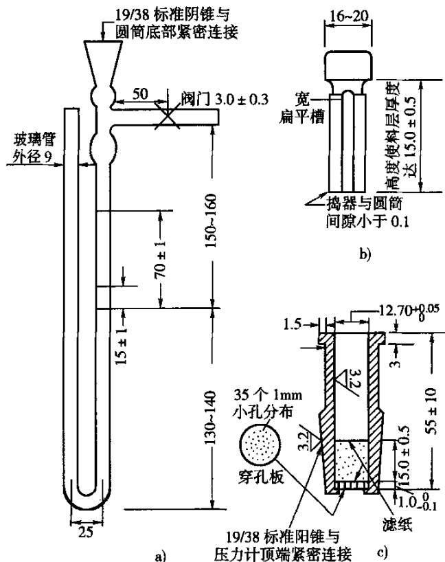
图 T0504-2 Blaine 透气仪结构及主要尺寸(尺寸单位:mm)
