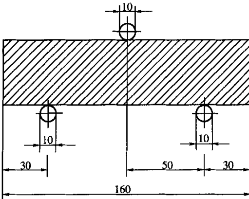
图 T0506-4 抗折强度测定加荷图(尺寸单位:mm)
